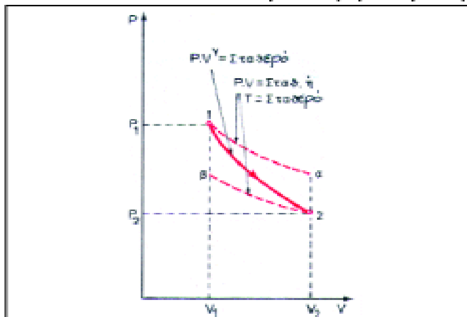
Εικόνα 1.1.4 Αδιαβατική μεταβολή
