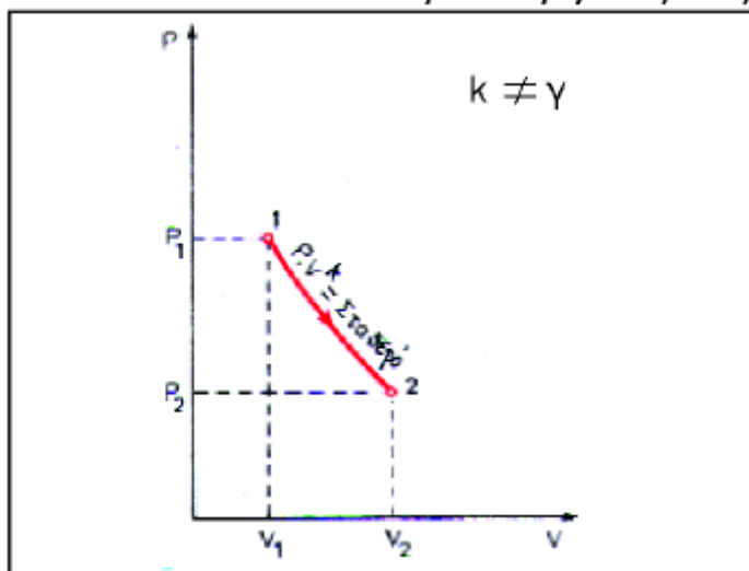
Εικόνα 1.1.5 Πολυτροπική μεταβολή
