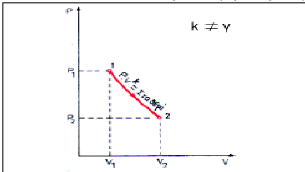
Εικόνα 1.1.5 Πολυτροπική μεταβολή
