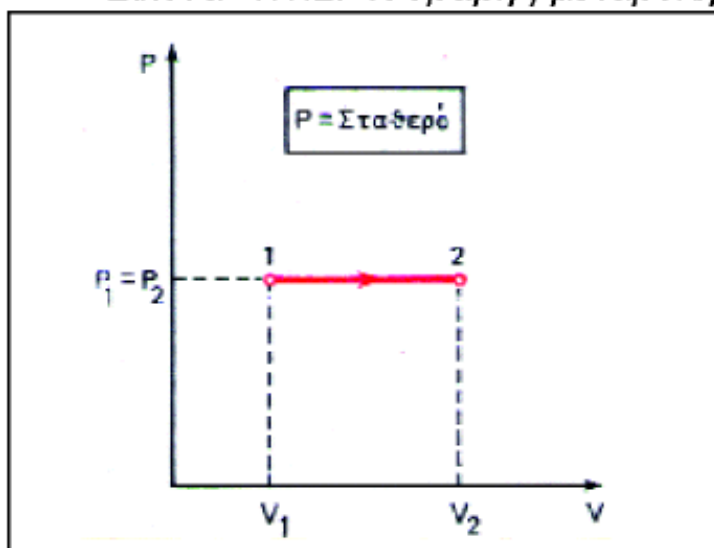
Εικόνα 1.1.2. Ισοβαρής μεταβολή
