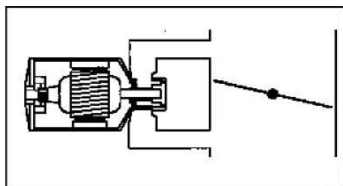
βαλβίδα αέρα με μοτέρ
