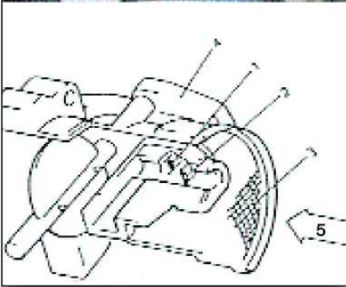
μετρητής μάζας MAF
