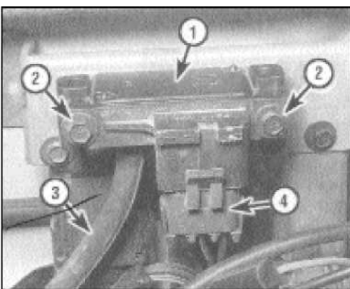
μετρητής απόλυτης πίεσης MAP
