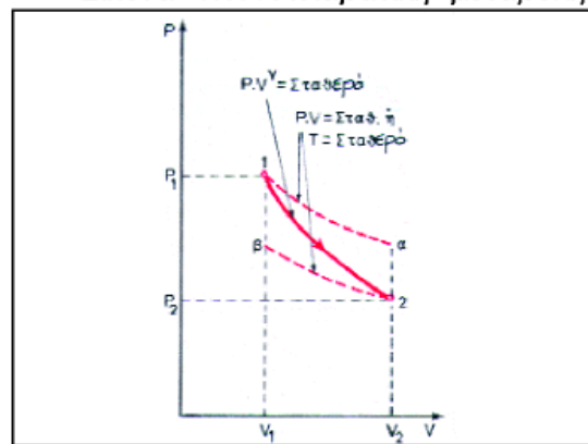
Εικόνα 1.1.5 Πολυτροπική μεταβολή
